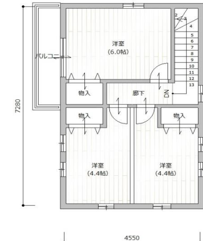
平面図 (2F)
