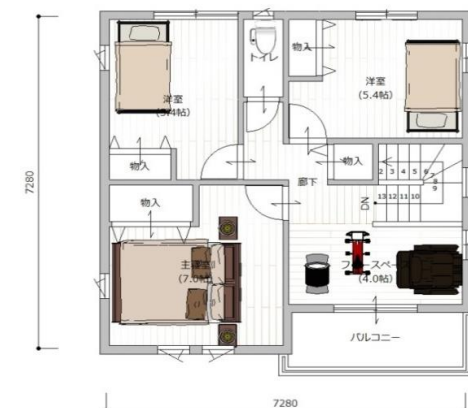
平面図 (2F)
